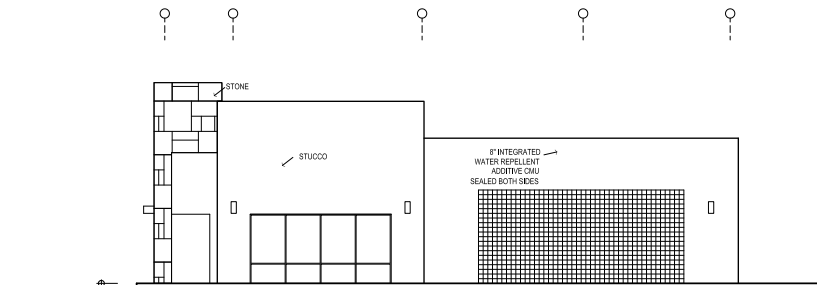
Right Elevation
